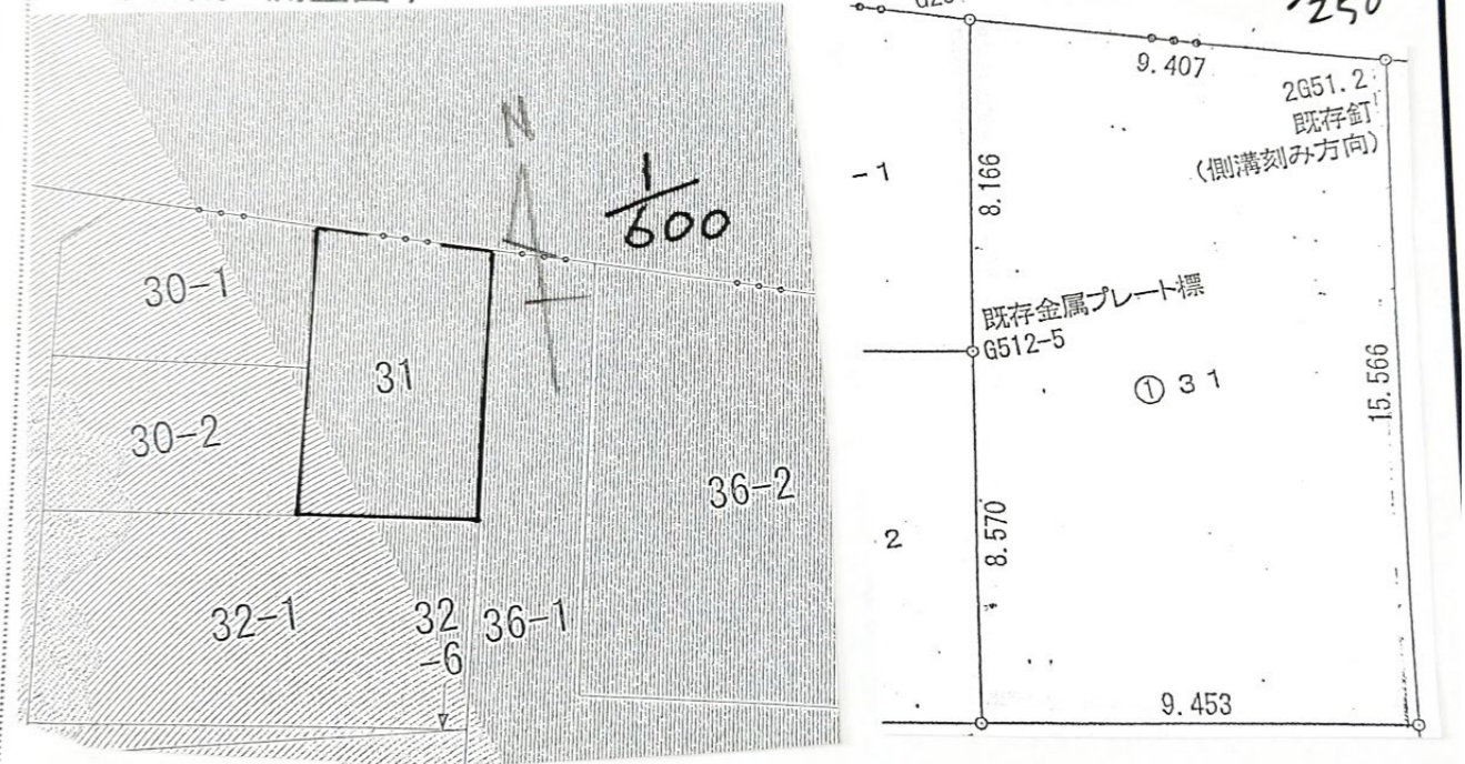
(公図・測量図)
